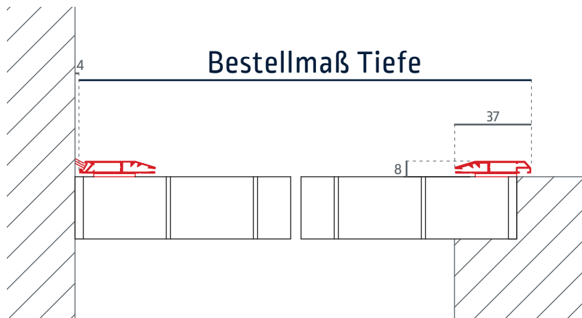
Befestigungsvariante mit Kautschukklebeband
